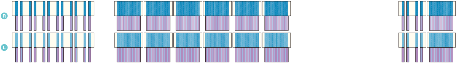
2000／N2000系気動車用カーテン(N用)[2101(TSE・量産化改造後)・プリーツカーテン] ×1
